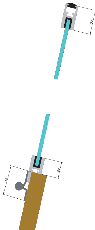
Doorsnede van boven- en onderprofiel
